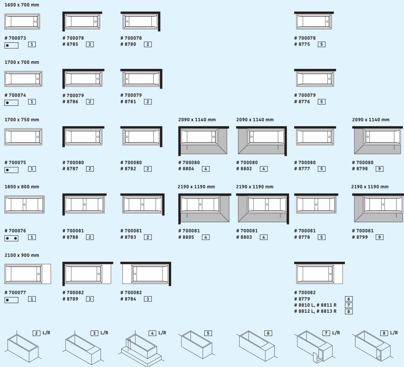
1 Badewanne Einbauversion, Bathtub Built-In, Vasca da bagno, versione da incasso, Baignoire à encastrer, Bad inbouwversie, Bañera accesorios de instalación no incluidos
